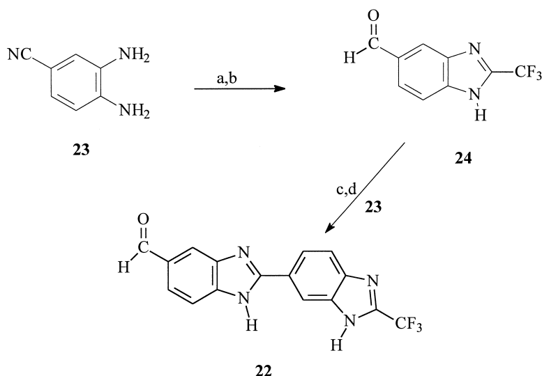
Scheme 3. (a) \text{CF}_3\text{COOH} , 90^\circ\text{C} ; (b) \text{HCOOH} , \text{NiAl (R)} ; (c) \text{PhNO}_2 , 145^\circ\text{C} ; (d) \text{HCOOH} , \text{NiAl (Ra-Ni)} .
